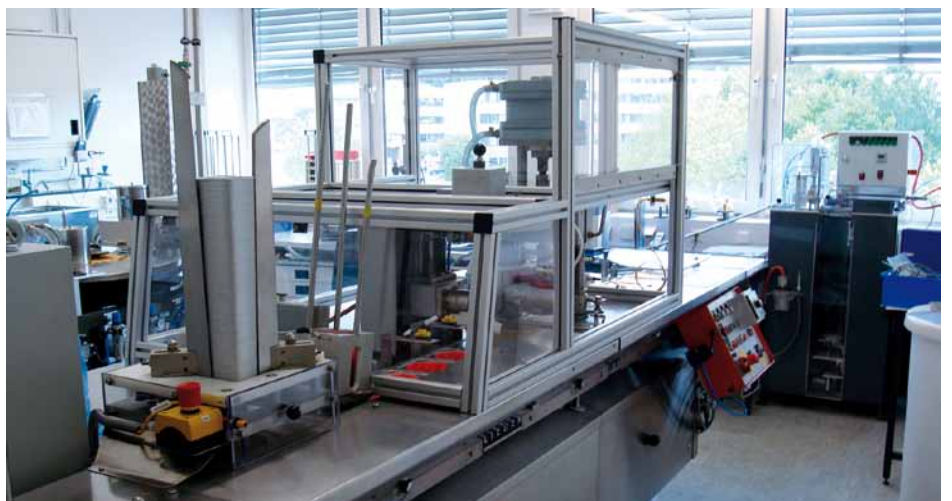
Siegelmaschine für die Pharmakonfektionierung u.a. mit komplett nachgerüsteten Sicherheitskomponenten
